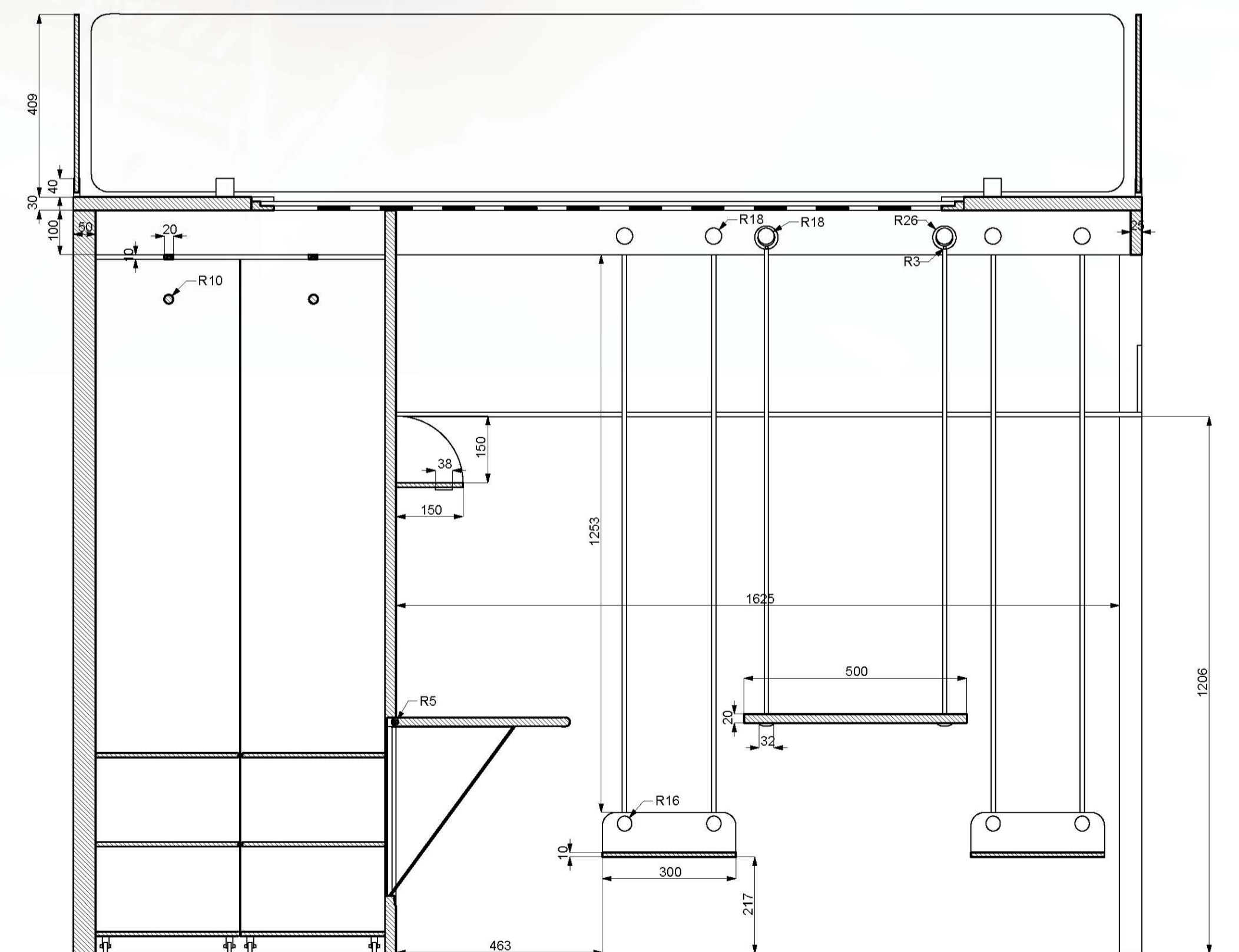
sezione B-B
