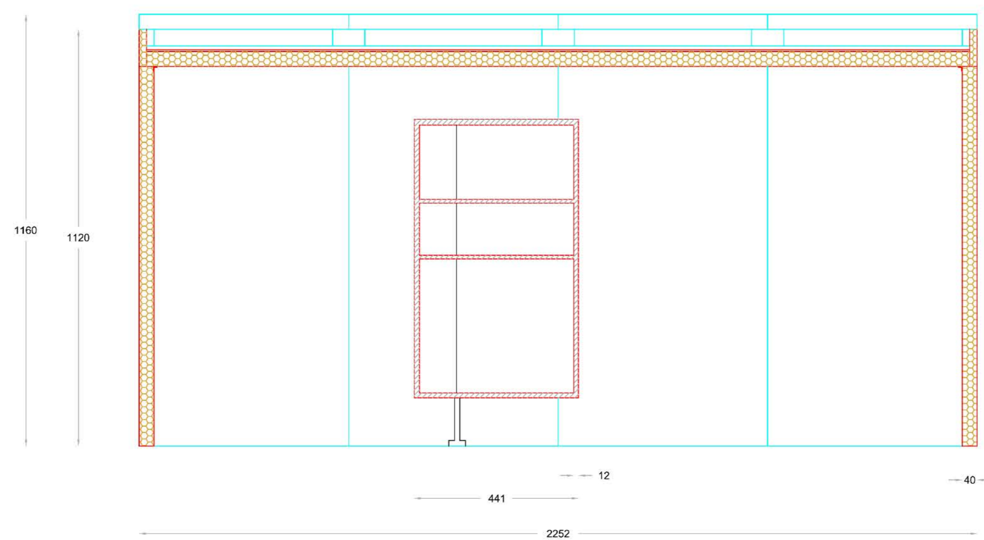
SEZIONE A - A'
