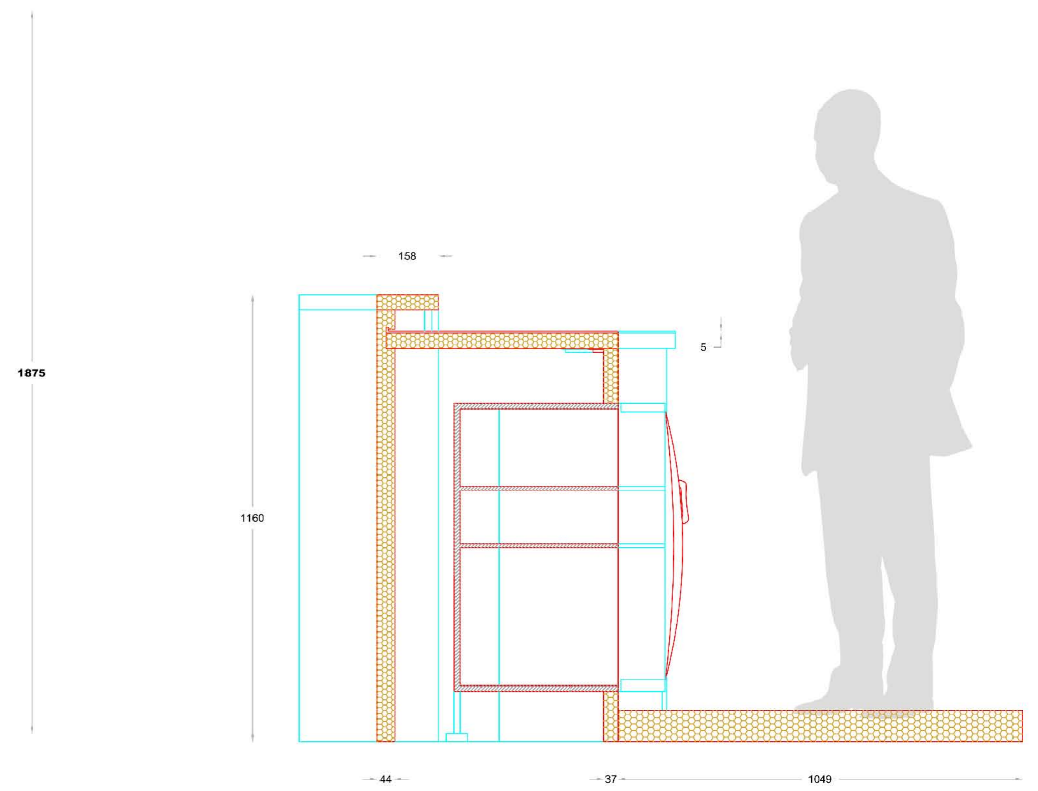
SEZIONE B - B'
