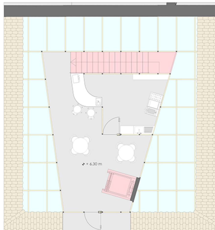
PIANTA LIVELLO 3 PARASSITA scala 1:50
