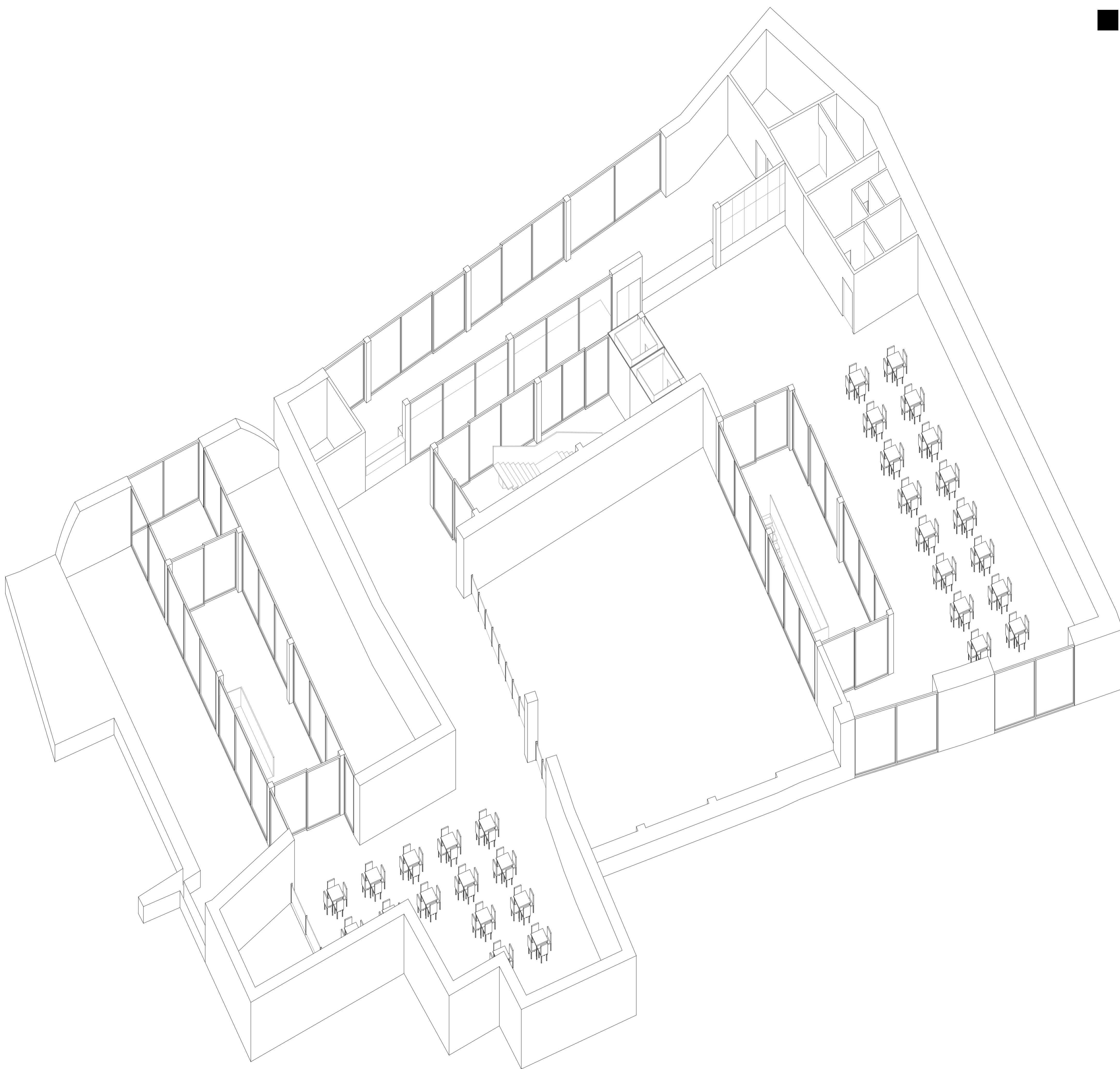
vista assometrica livello ristorante _ scala 1:200
