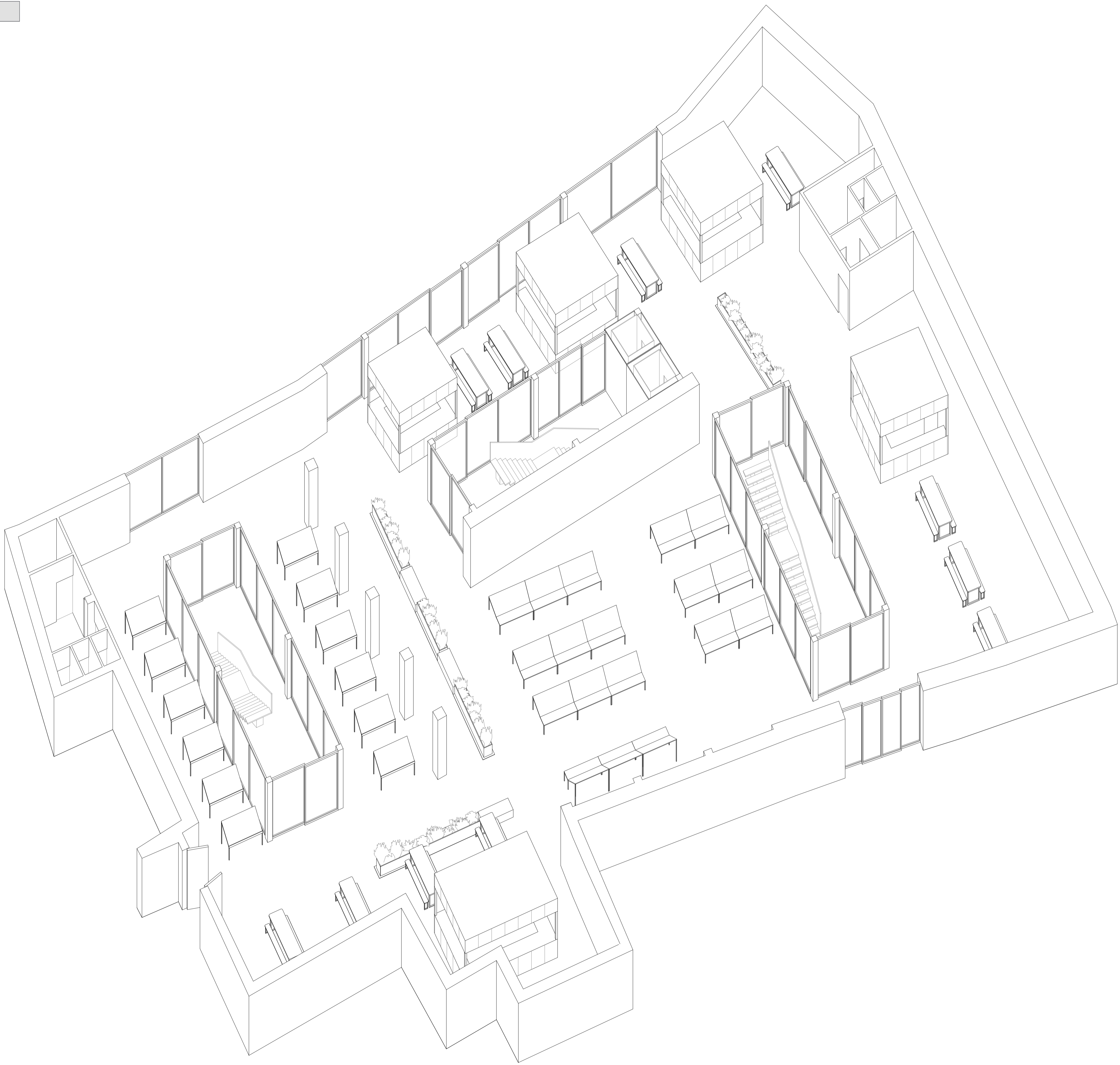
vista assonometrica livello mercato ortofrutticolo e slow food _ scala 1:100
